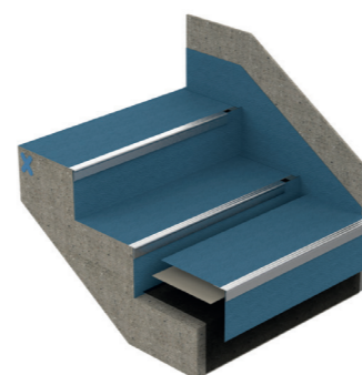
TRIFLEX TSS SYSTEEM, 3-LAAGS
